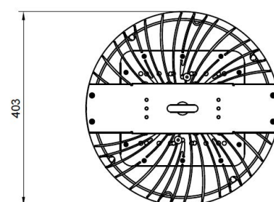
UKKO 100/145
